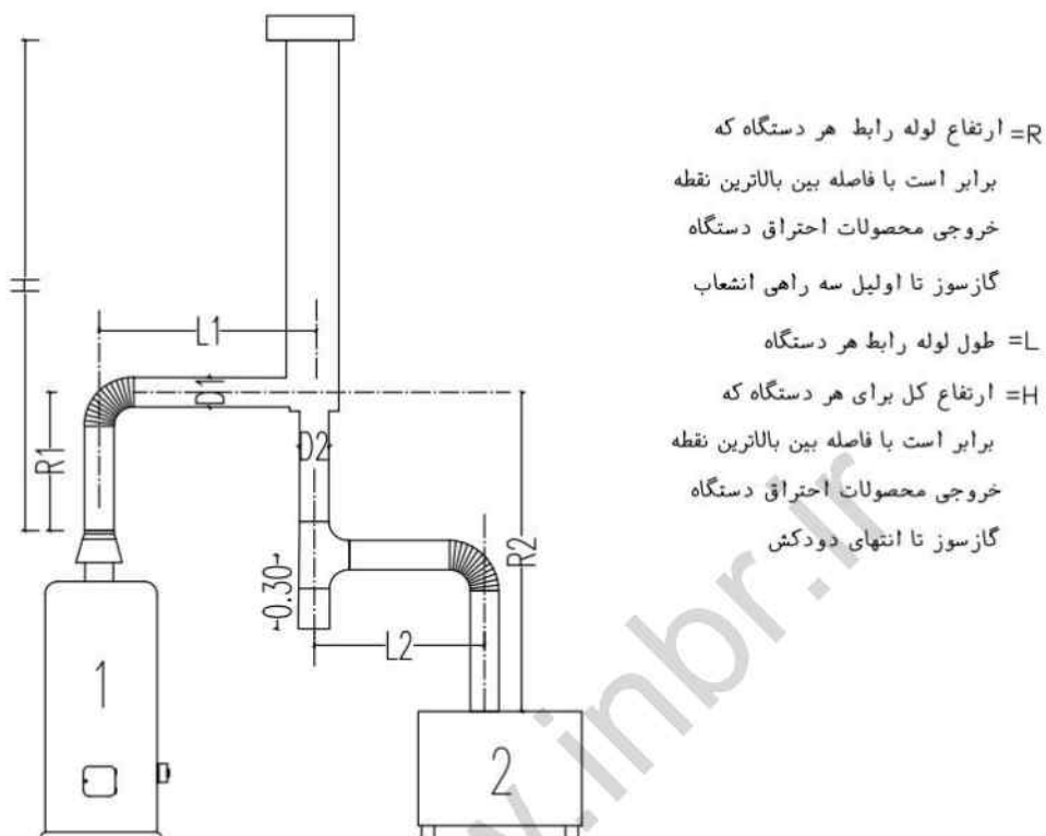
شکل ۴-۱۷-۲ دودکش برای دو یا چند دستگاه گازسوز که در یک طبقه نصب شده‌اند
